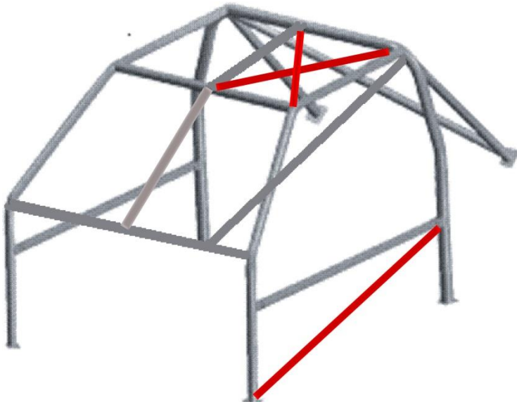
Voorbeeld kooiconstructie:
